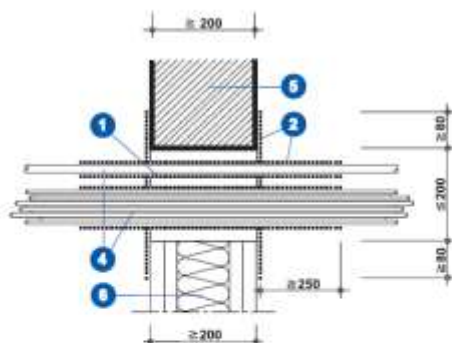
Detalj B - Protupož. zapreka kod kabela bez dodatnih trakica
